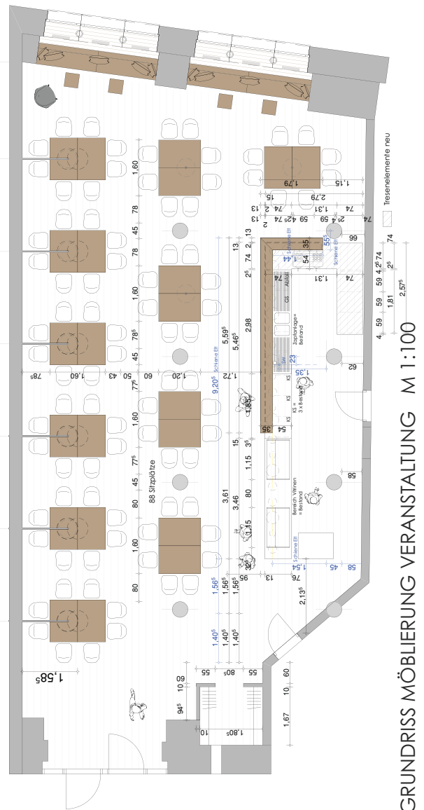
GRUNDRISS MÖBLIERUNG M 1:100
